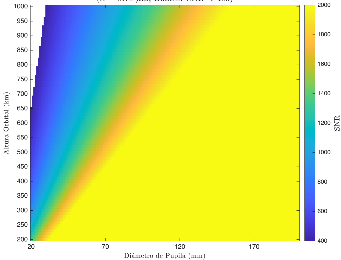
SNR - Refractivo - Detector 2 ( \lambda = 0.76 \mu\text{m} , Blanco: SNR < 400)
